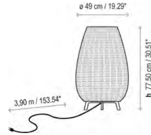
Amphora 01 IP-66
